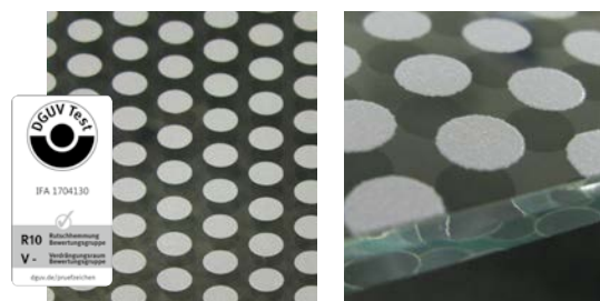
Rutschhemmungsklasse R10 als Punkte-Dekordruck; Bedruckungsgrad 40 %, Punkte 8 mm
