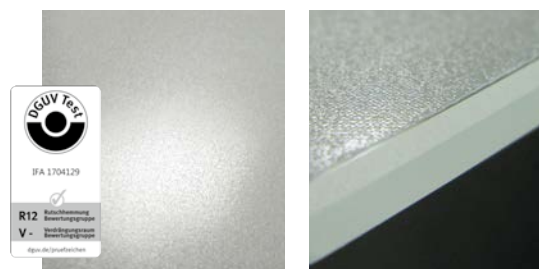
Rutschhemmungsklasse R12 als vollflächige Ätztön-Bedruckung
